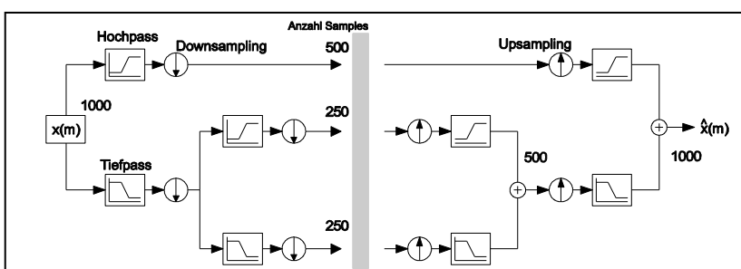
Schnelle Wavelet Transformation
